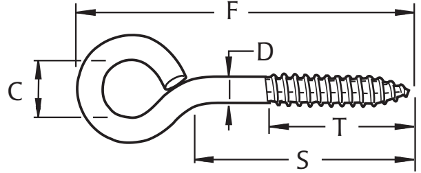
Eye Bolt (Lag Tread)
